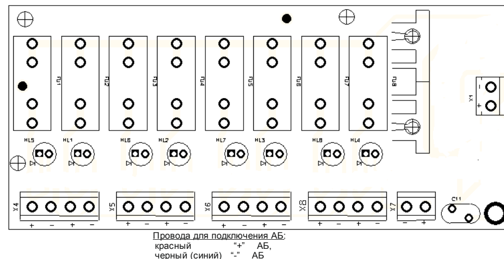
Рис. 1. Схема подключения УЗК-8Р
